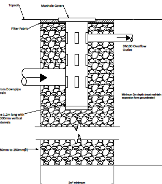
SECTION A Scale: 1:10 @ A1
